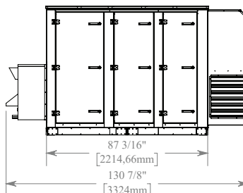
Devant/Front
